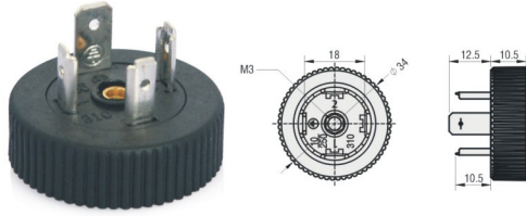
A型圆形螺纹安装插座
