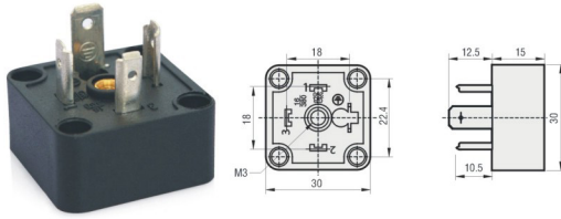
A型仪表表插座
