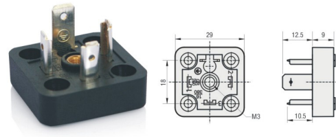
A型插座, 方形 四个固定孔
